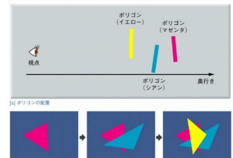
■ 図4.6—奥行きソート法の描画過程
